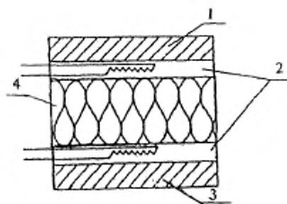
Рисунок А.2 — Схема прибора с двумя тепломерами
