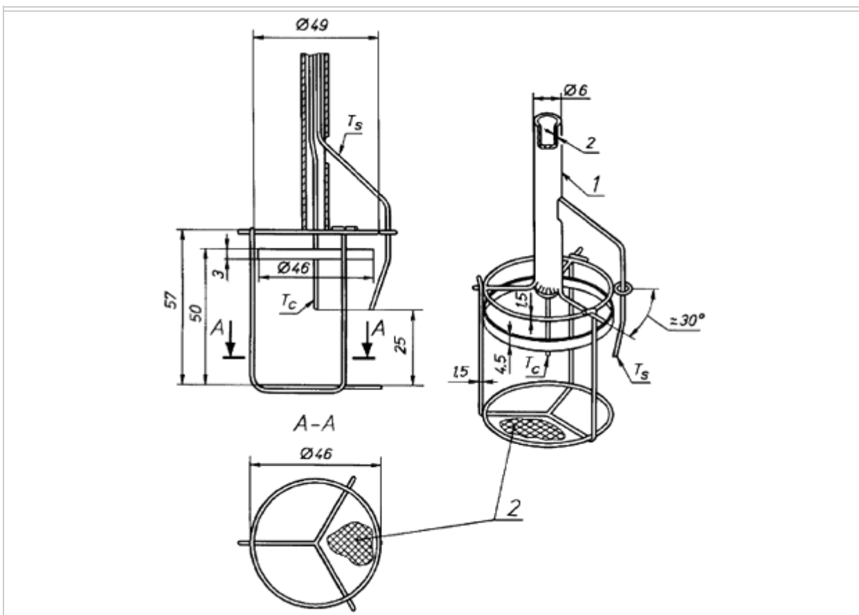
Рисунок А.2 - Обмотка печи
