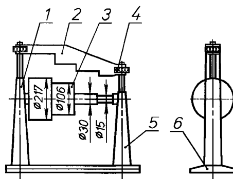
1 — опора; 2 — прижимная планка; 3 — цилиндр; 4 — гайка; 5 — опора; 6 — основание
