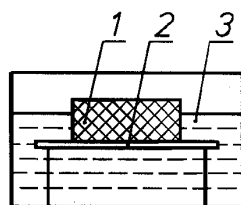
1 — образец; 2 — сетчатая подставка; 3 — ванна с водой
