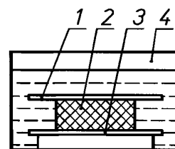
1 — сетчатый пригруз; 2 — образец; 3 — сетчатая подставка; 4 — ванна
